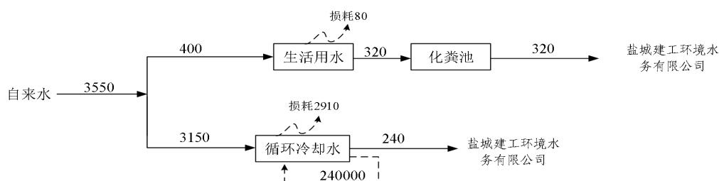
图 2-1 水平衡图 (单位: \text{t}/\text{a} )
